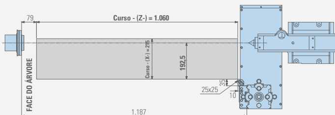
Torneamento externo
