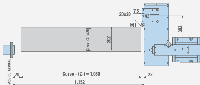
Torneamento externo
