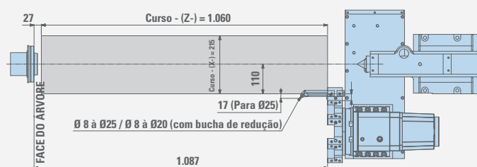
Torneamento interno
