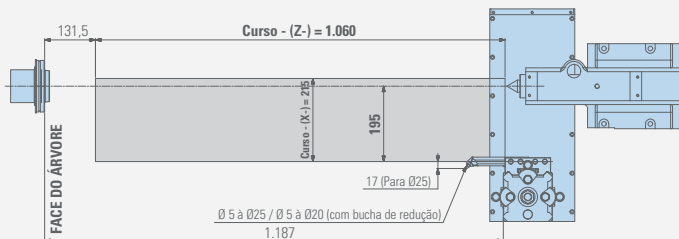
Torneamento interno
